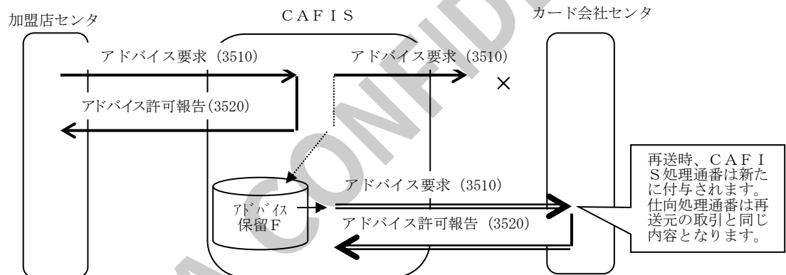
図 3.3-7 被仕向センタ送信異常
