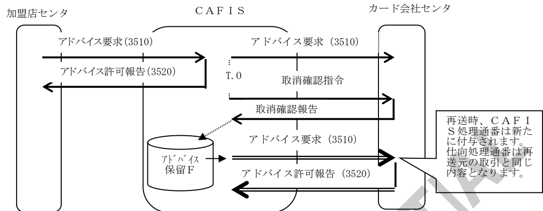
図 3.3-6 被仕向センタタイムアウト
