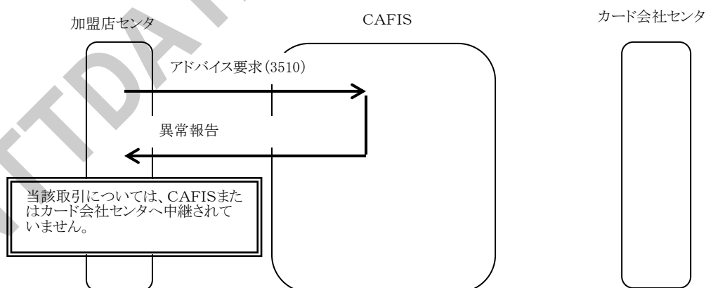
図 3.3-13 CAFISセンタ異常報告応答
